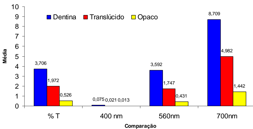
Gráfico 1: Médias de porcentagem de T direta para o espectro (%T) e nos comprimentos de onda de 400, 560 e 700 nanômetros para as cores Dentina, Translúcido e Opaco da resina composta Charisma
