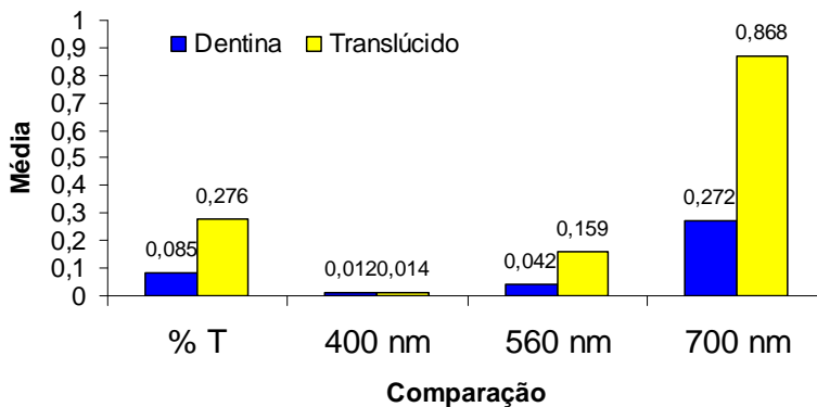
Gráfico 3: Médias de percentagem de Td para o espectro (%T) e nos comprimentos de onda de 400, 560 e 700 nanômetros para as cores Dentina e Translúcido da resina composta Intens
