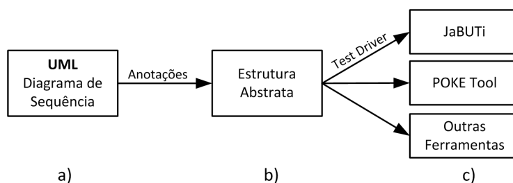
Figura 2. Abordagem para a geração de casos de testes estrutural
