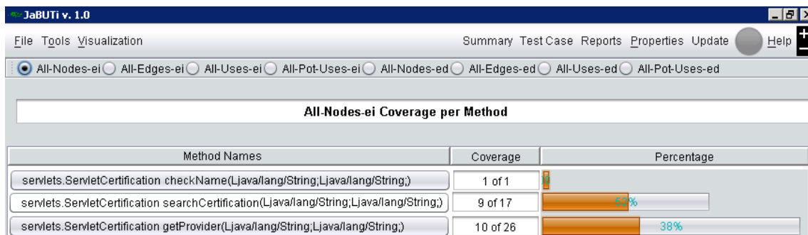
Figura 8. Interface da JaBUTi com as informações de cobertura dos métodos testados
