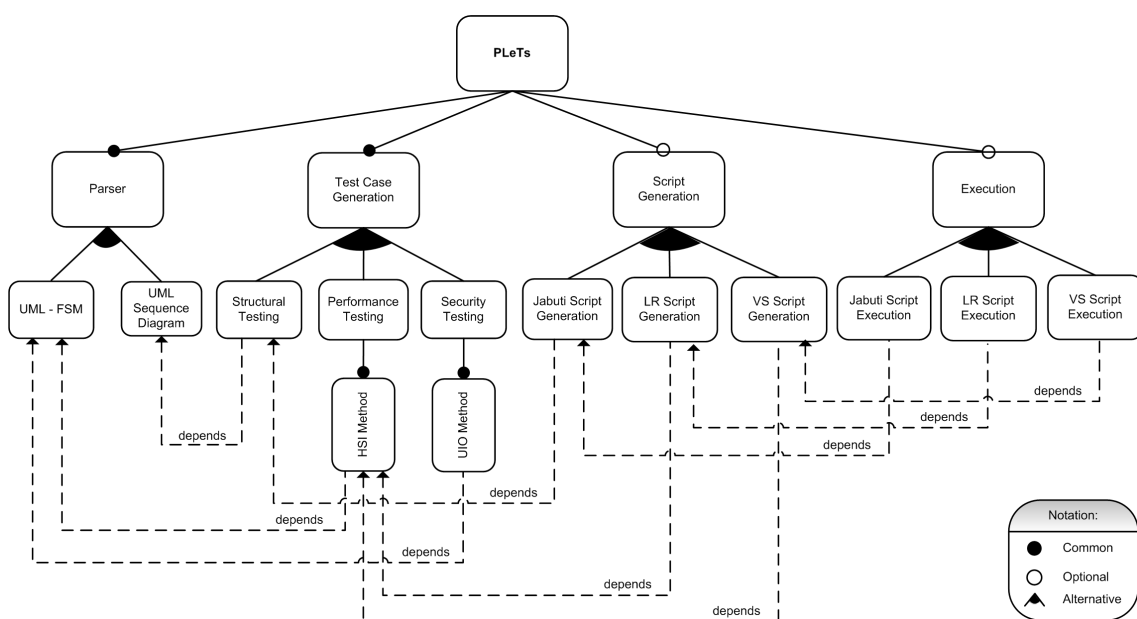
Figura 1. Modelo de características da PLeTs PL [Rodrigues et al. 2010]
