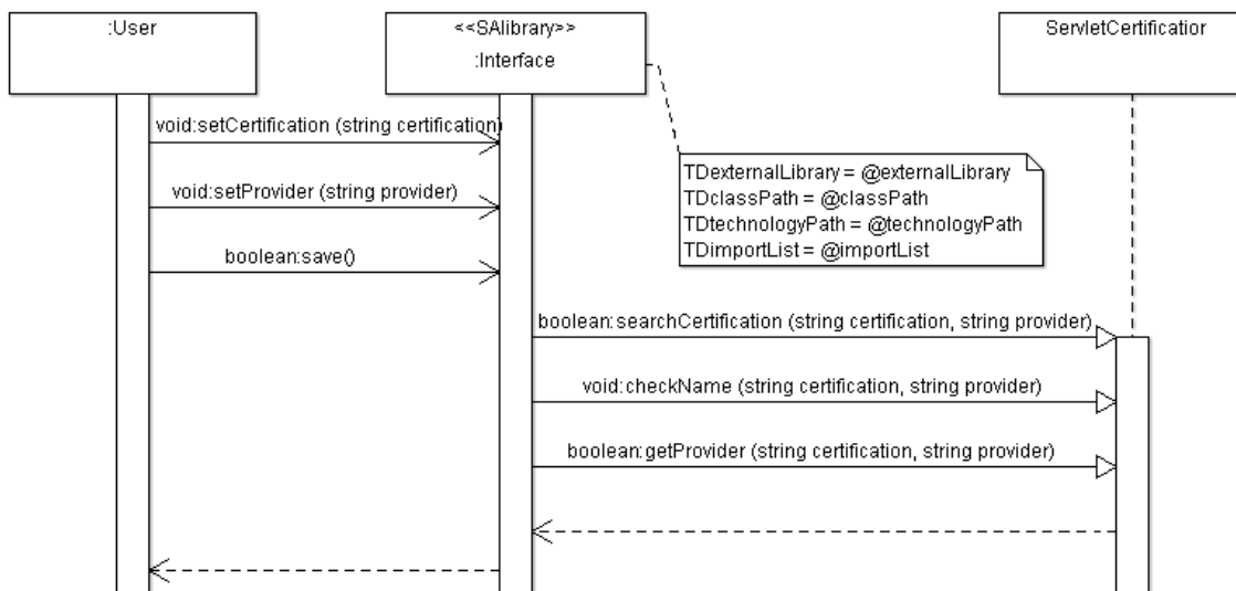
Figura 3. Diagrama de sequência para busca de certificação
