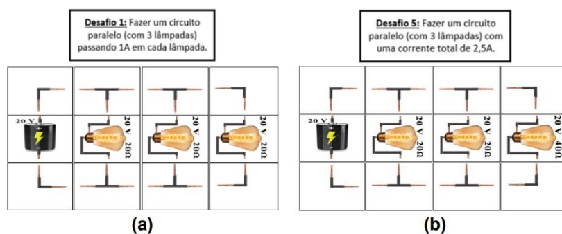
FIGURA 4 Circuitos completos do Desafio 1 (a) e do Desafio 5 (b) Elaborado pelos Autores
