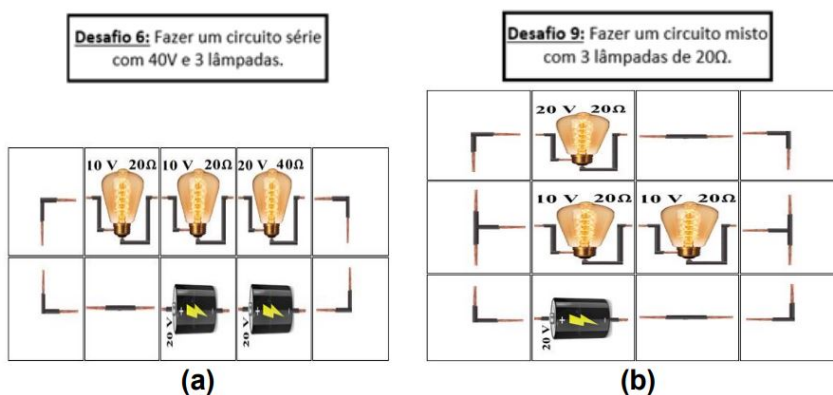
FIGURA 5 Circuitos completos do Desafio 6 (a) e do Desafio 9 (b) Elaborado pelos Autores
