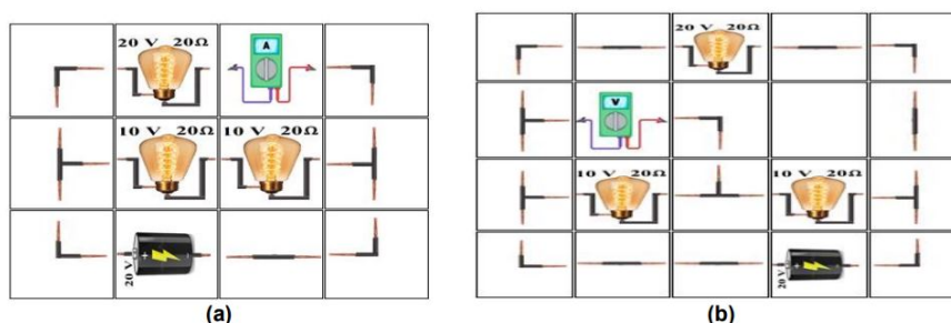
FIGURA 7 Circuito do Desafio 9 com a inserção de um amperímetro (a) e de um voltímetro Elaborado pelos Autores
