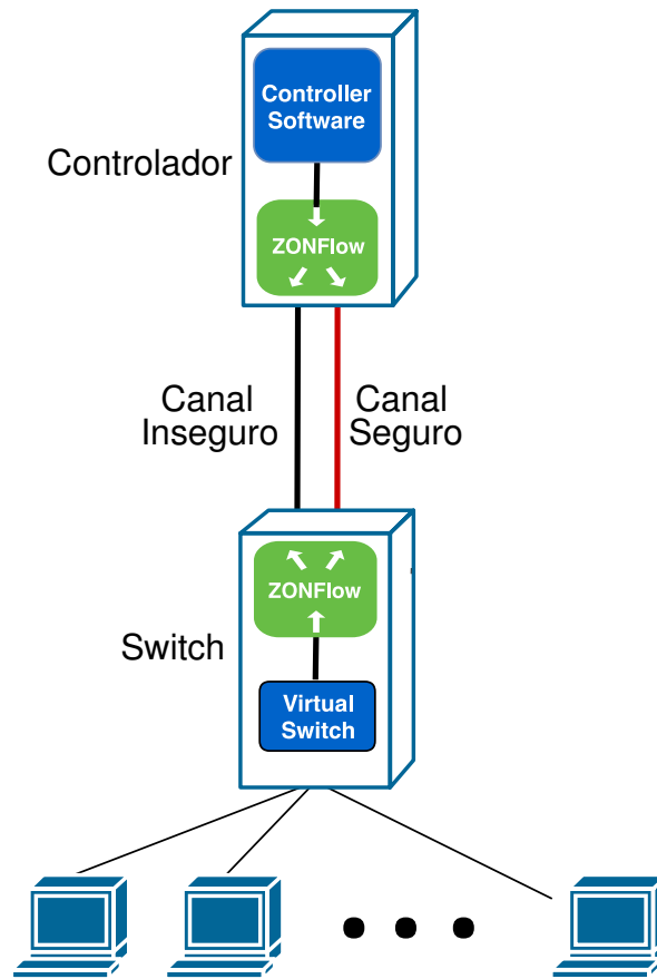
Figura 4.2 – Arquitetura ZONFlow.
