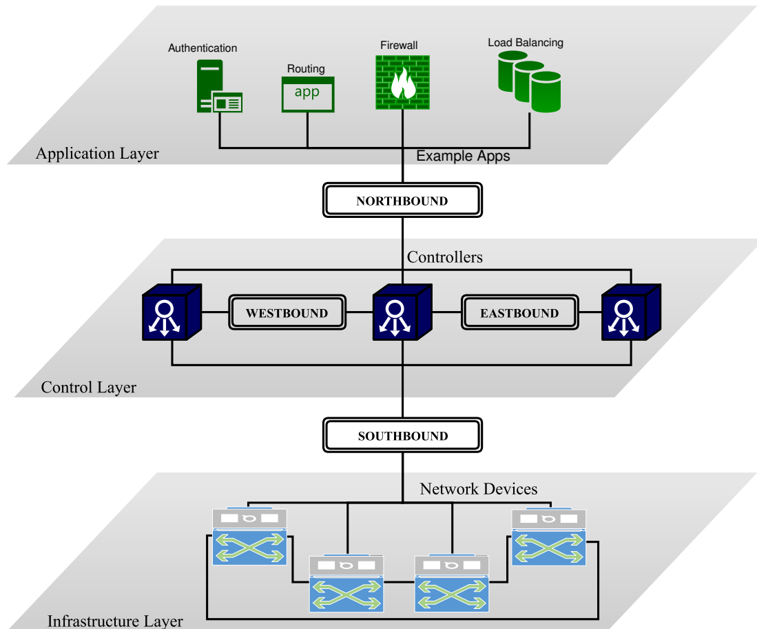
Figura 2.4 – Arquitetura SDN
