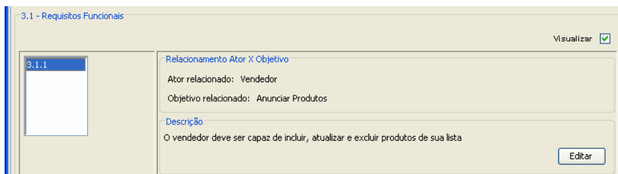
Figura 23 – Requisito modificado conforme execução da regra.
