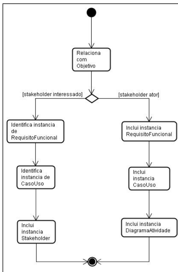
Figura 46 – Diagrama de atividades: inclusão da instância de Stakeholder.
