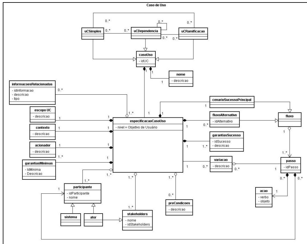
Fig. 3 - Modelo Conceitual dos Casos de Uso
