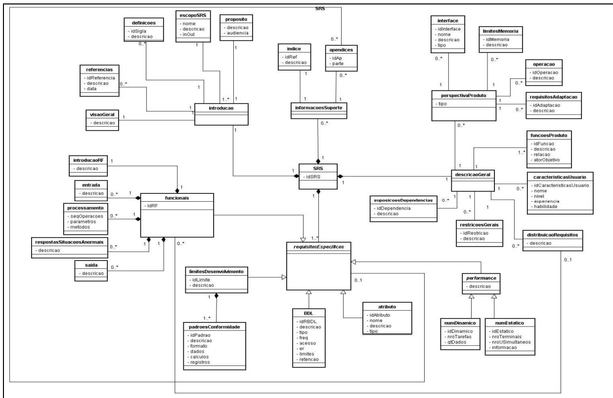
Fig. 2 – Modelo Conceitual da SRS.
