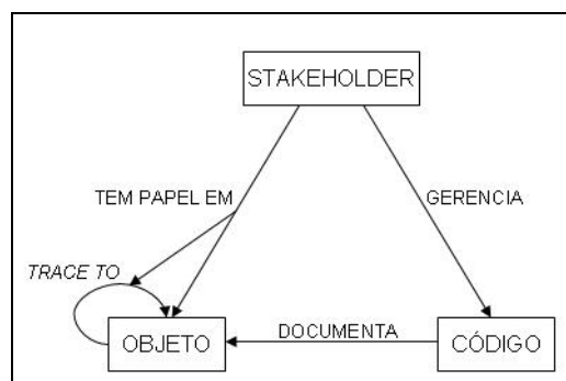
Figura 15 – Metamodelo de rastreabilidade (adaptado de [RAM01]).
