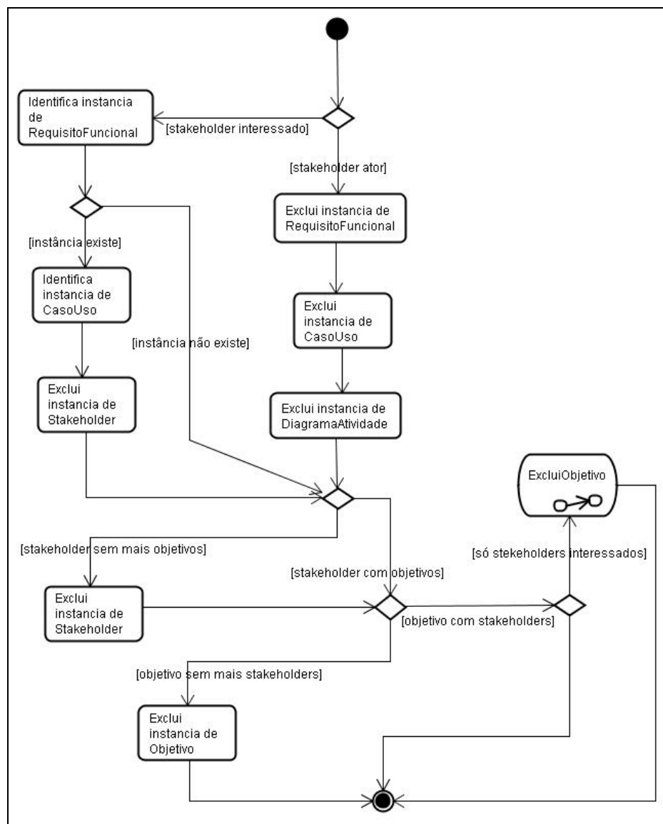
Figura 39 – Diagrama de atividades: exclusão de um relacionamento.
