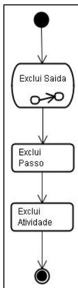
Figura 34 – Diagrama de atividades: exclusão da instância de Processamento.
