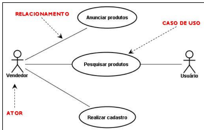
Figura 8 – Diagrama de caso de uso.
