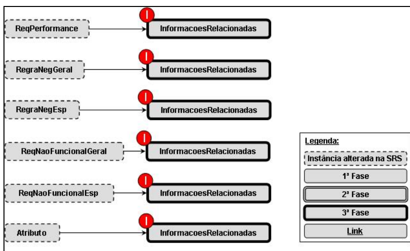
Figura 27 – Classes impactadas quando da substituição das instâncias de RegraNegGeral, RegraNegEsp, ReqNaoFuncionalGeral, ReqNaoFuncionalEsp, ReqPerformance, Atributo.
