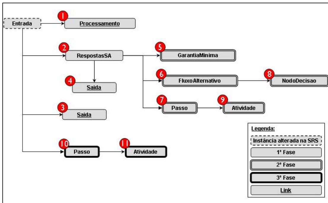
Figura 29 – Classes impactadas quando da substituição de uma instância de Entrada.
