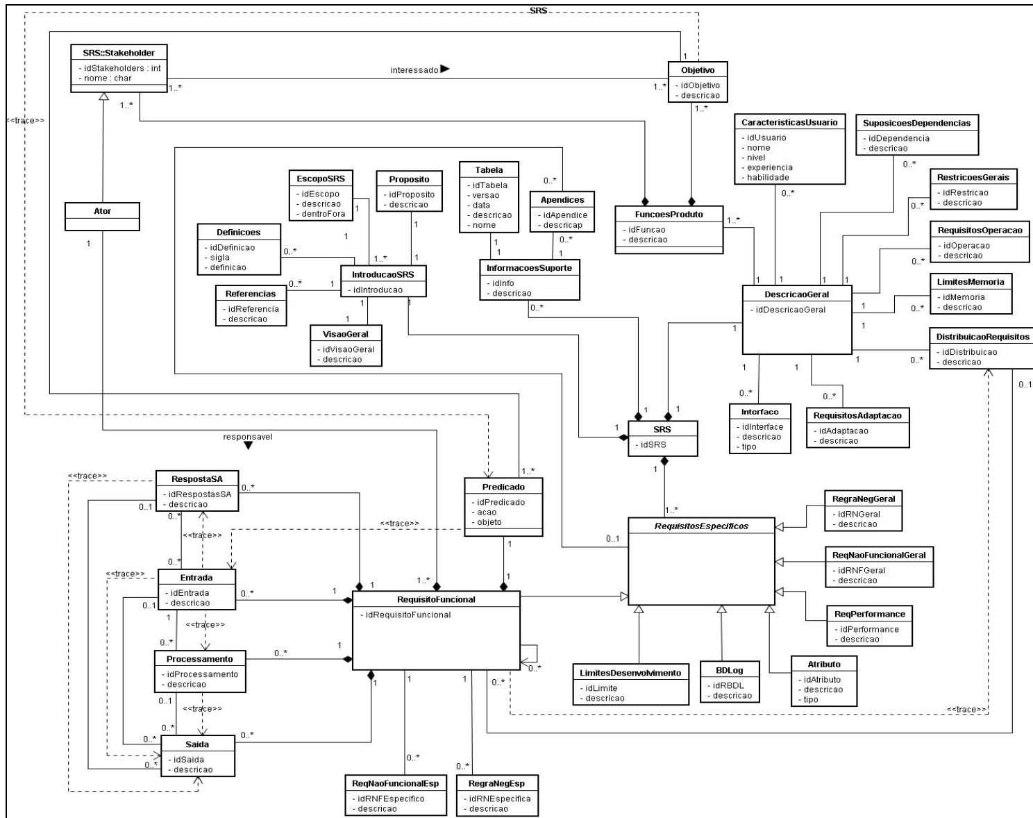
Figura 22 – Modelo conceitual da SRS.
