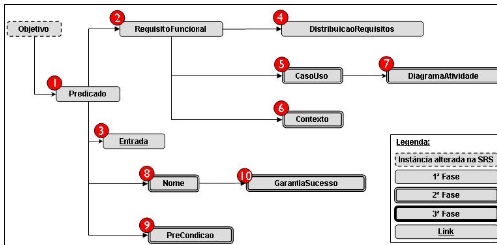
Figura 31 – Classes impactadas quando da substituição de uma instância de Objetivo.
