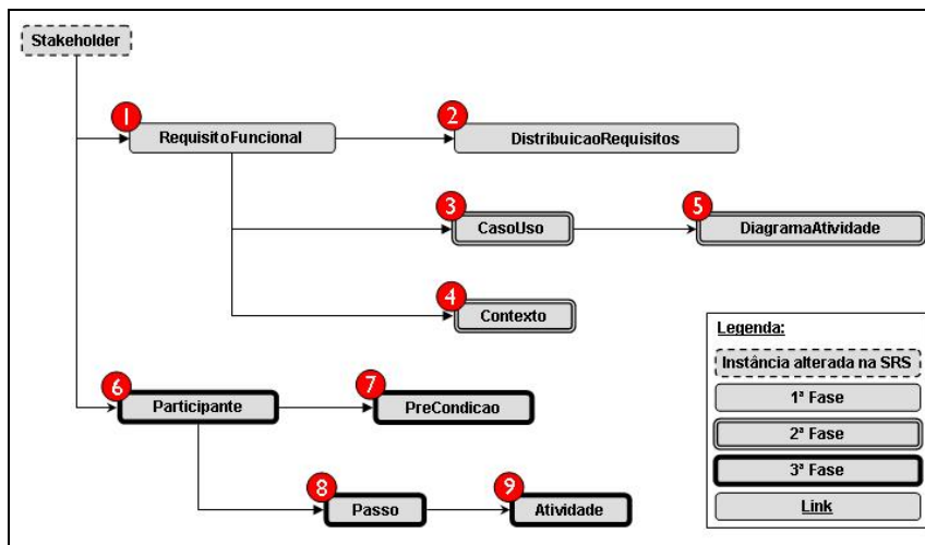
Figura 30 – Classes impactadas quando da substituição do stakeholder.
