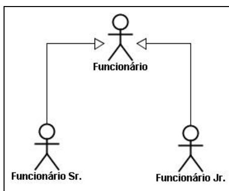
Figura 9 – Generalização de atores.
