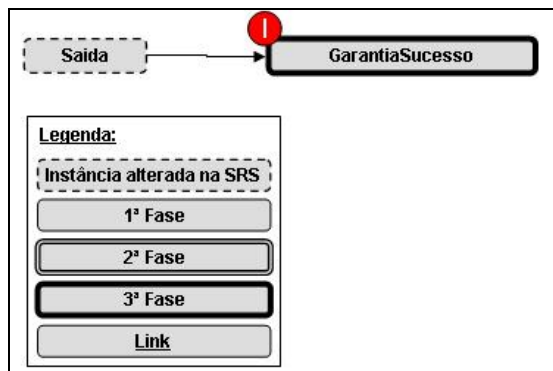
Figura 26 – Classes impactadas quando da substituição de uma instância de Saida.
