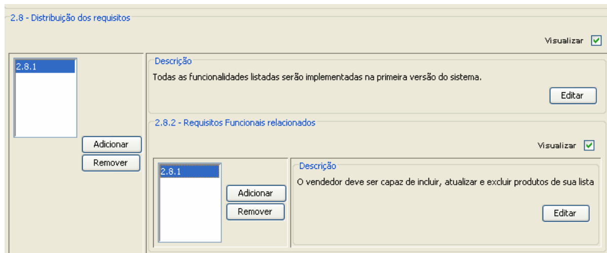
Figura 24 – Requisitos ligados à seção DistribuicaoRequisitos.
