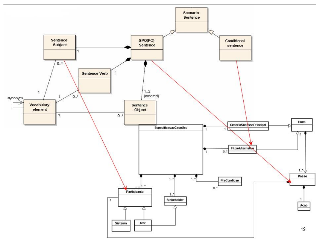
Figura 23 – Relação do metamodelo de [SMI05] com o modelo conceitual do MCU.
