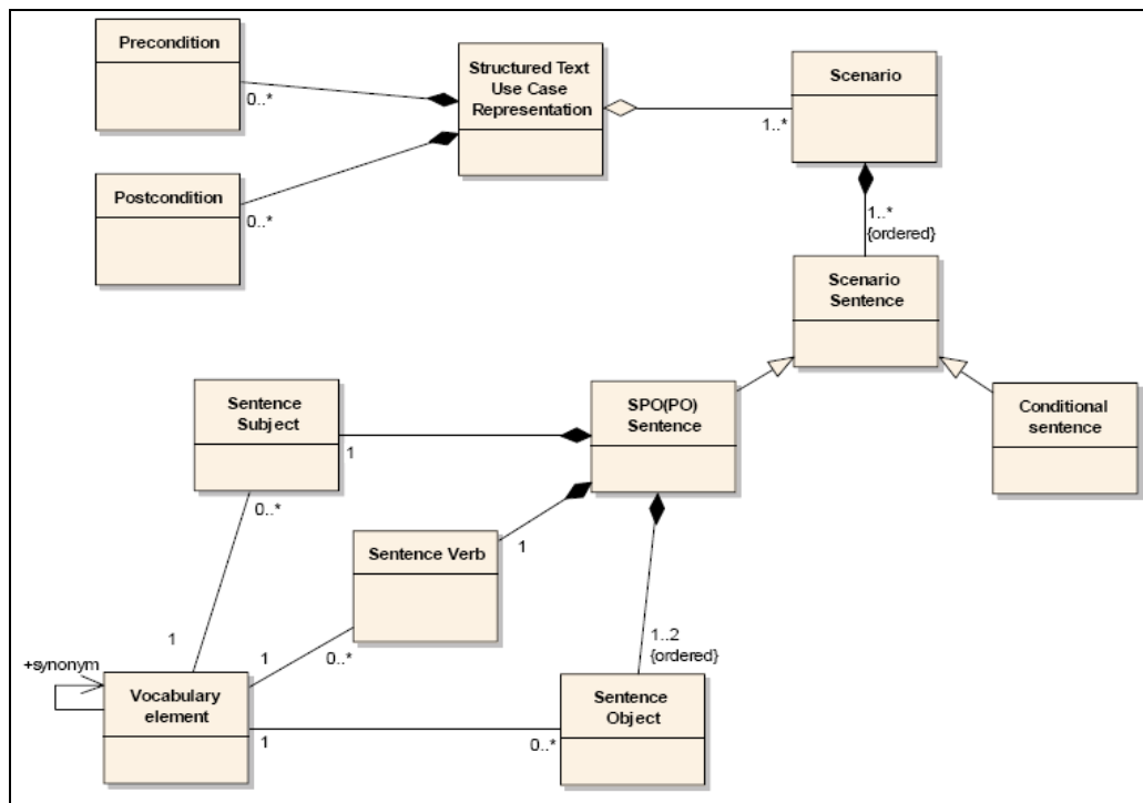
Figura 12 – Metamodelo para representação textual estruturada [SMI05].
