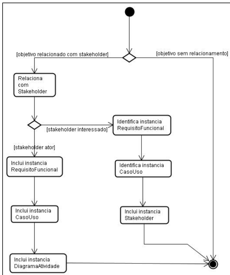
Figura 47 – Diagrama de atividades: inclusão da instância de Objetivo.
