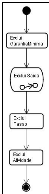
Figura 35 – Diagrama de atividades: exclusão da instância de RespostasSA.
