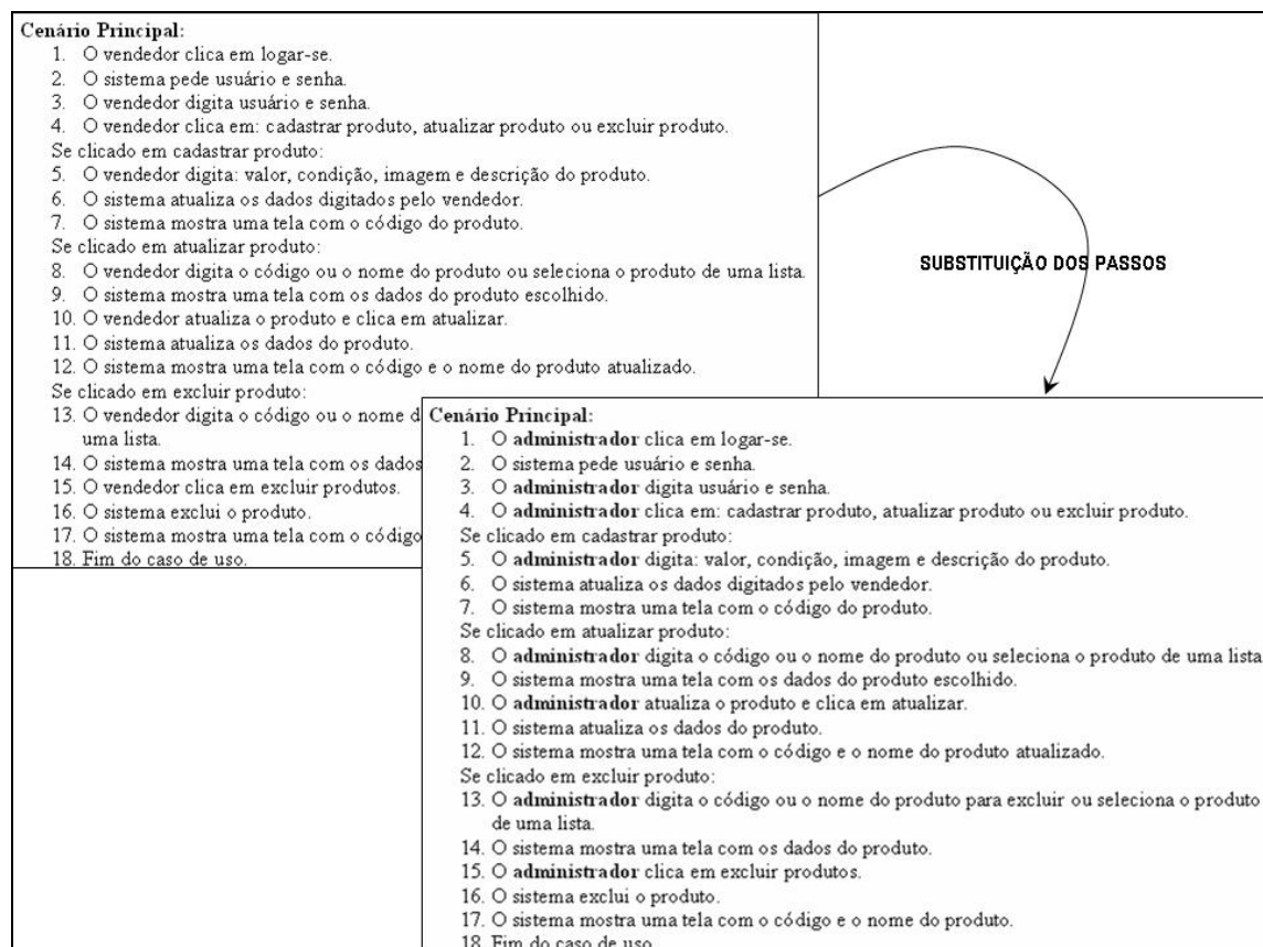
Figura 52 – Alteração dos passos conforme substituição do participante.
