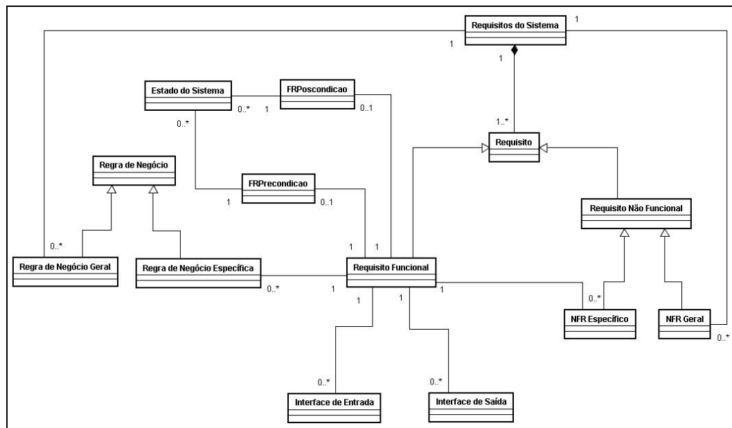
Figura 2 – Meta-modelo de requisitos.
