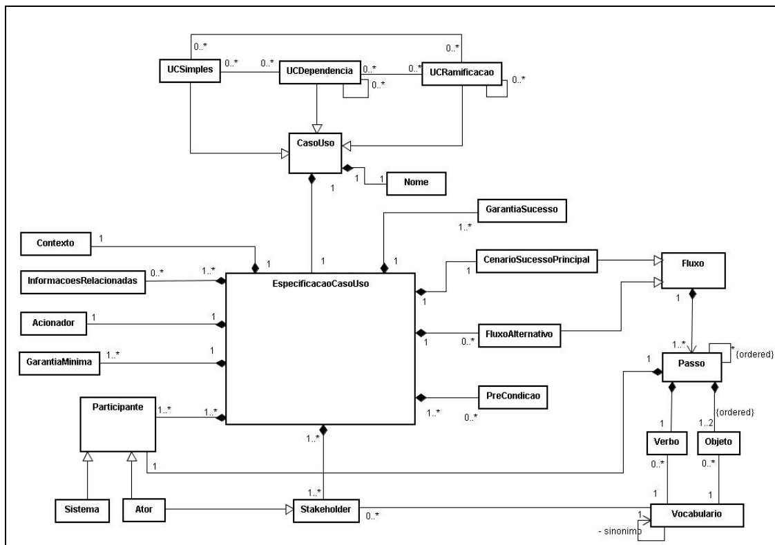
Figura 24 – Modelo conceitual do MCU adaptado.
