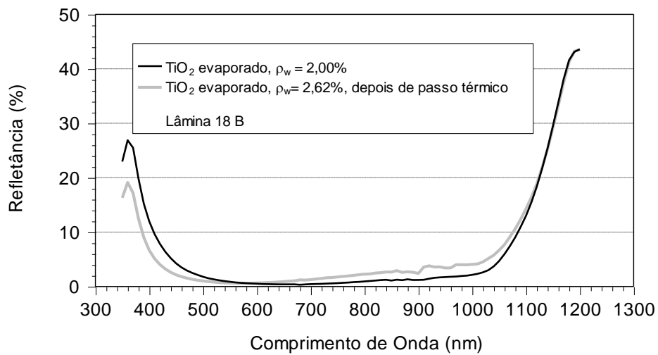
Figura 6 - Refletância espectral de filme de \text{TiO}_2 depositado por evaporação, antes e depois do processo térmico a 840\text{ }^\circ\text{C} . Medida realizada no ponto central da lâmina (ponto 1).
